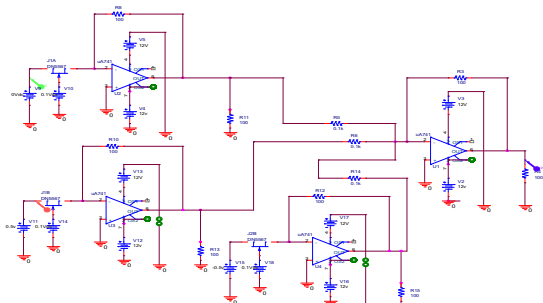
図2 基本的なニューロンモデル (アナログ電子回路を使用し、ニューロンの結合係数は乗算回路により実現しています。多数組み合わせることで深層学習の基本モデル実現も目指しています)
