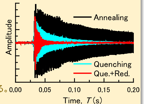
チタン合金の減衰曲線の変化
