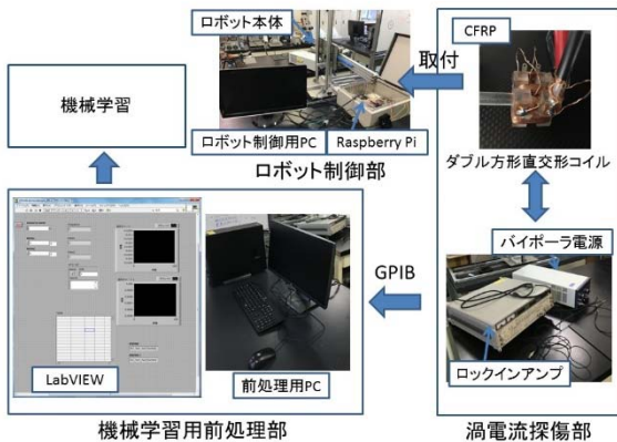
機械学習を用いた複合材の渦電流非破壊検査ロボットシステム
