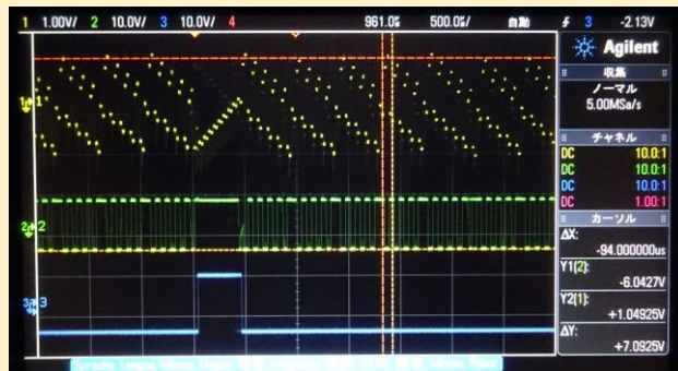
左の回路で観測された電荷平衡型+シングルスロープ型A/D変換の波形
