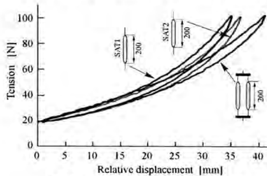
図10 並列接続(初期張力 = 20[N])
