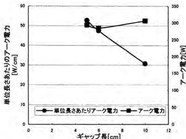
図9 電極間上部3cmに石英ガラス板を設置した場合の アーカ電力の変化
