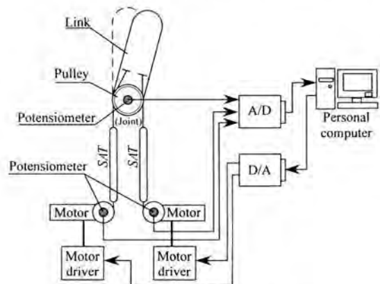
図 13. 一関節ロボットの構成
