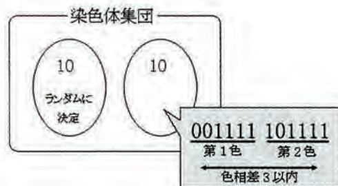
図4.2 初期集団の生成
