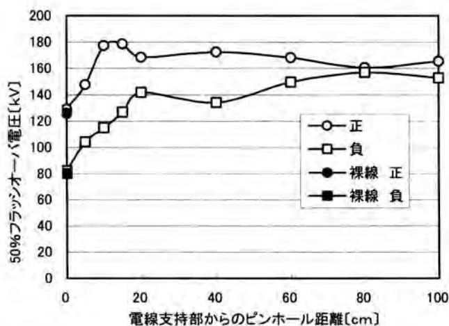
図3. ピンホルル位置による50%フラッシュオーバー電圧の変化
