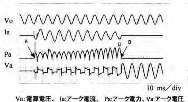
図2 アーク発生時の電源電圧、アーク電圧、アーク電流およびアーク電力の各波形例
