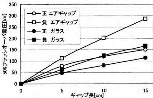
図8. ギャップ長を変化させた場合の50%フラッシュオーバー電圧
