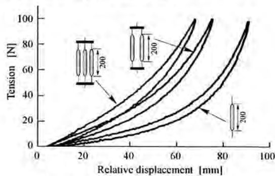
図9 並列接続(初期張力 = 0 [N])
