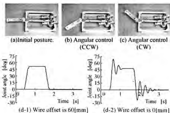
図 16 関節角度の制御
