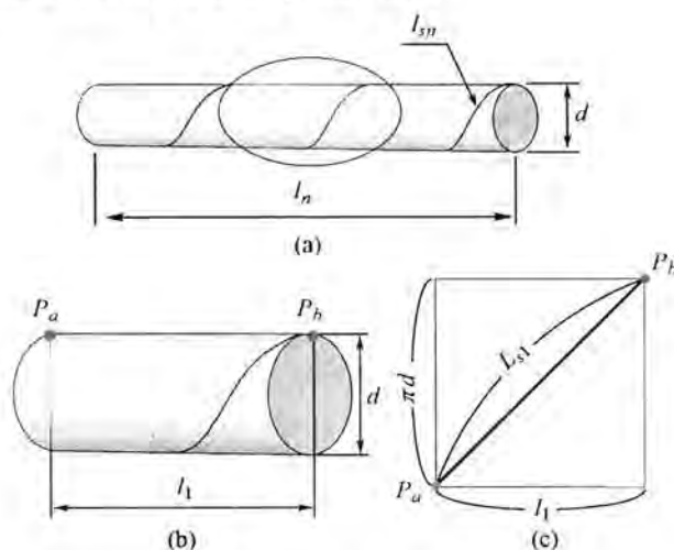
図 3 SAT の幾何学的モデル化
