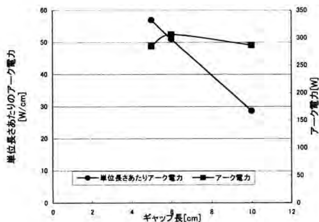
図8 電極間上部0cmに石英ガラス板を設置した場合の アーカ電力の変化
