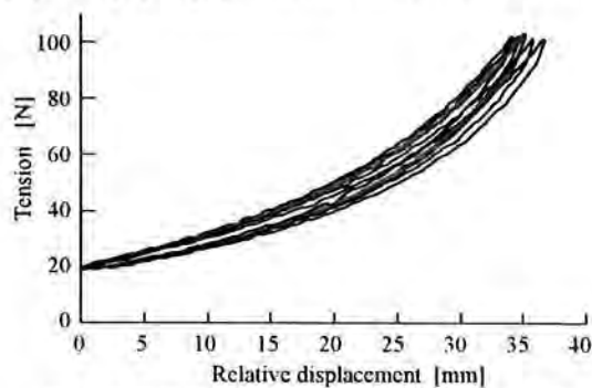
図7 SATの静特性(個体間の特性のバラツキ)
