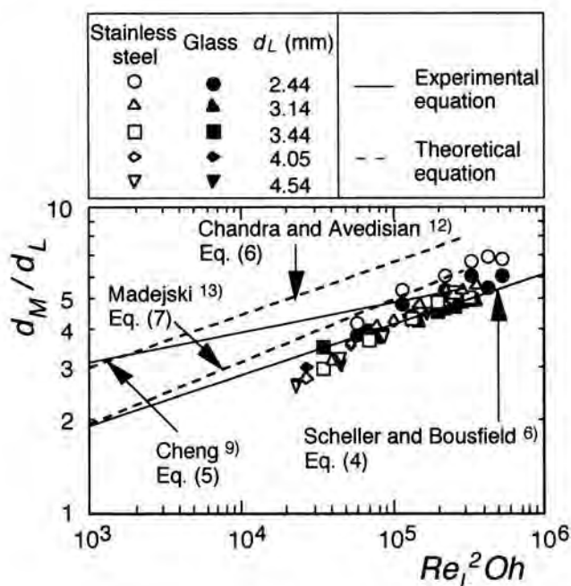
図10 無次元数 Re_L^2 Oh による 最大直径比 d_M/d_L の整理
