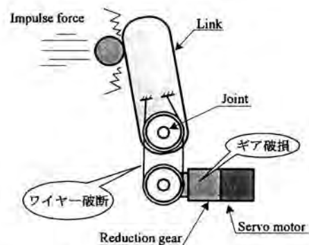
図1 機構的に硬い動力伝達機構の問題点
