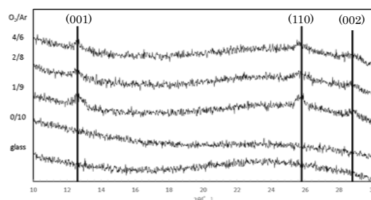
図 3 \text{VO}_x 薄膜の XRD スペクトル
