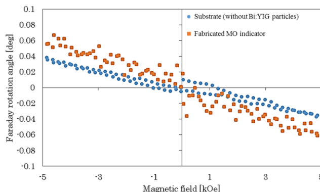
図3 作製したMOセンサのMO効果測定結果
