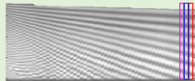
オイルフィルム法を用いた 壁面せん断応力の測定
